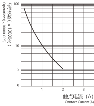
电耐久性曲线 ENDURANCE CURVE
